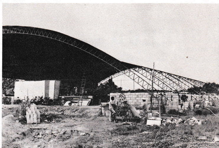
Vista da obra do Núcleo Educacional.
